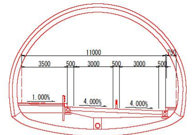
トンネル部標準断面図
