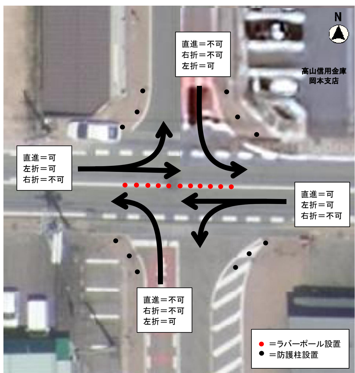
詳細図
