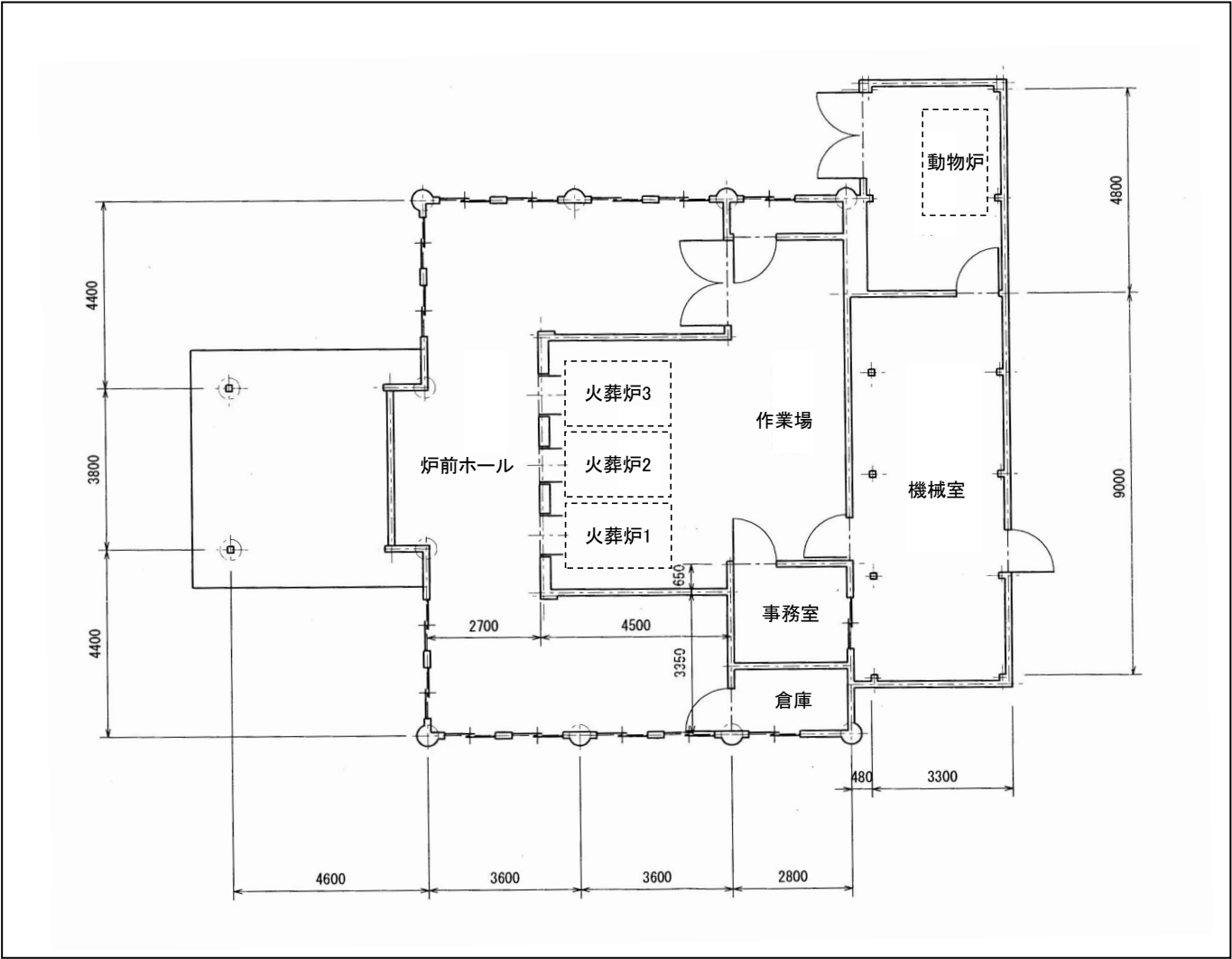
現施設火葬棟平面図
