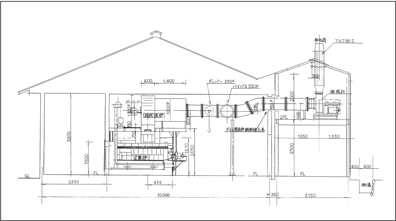
現施設火葬棟断面図
