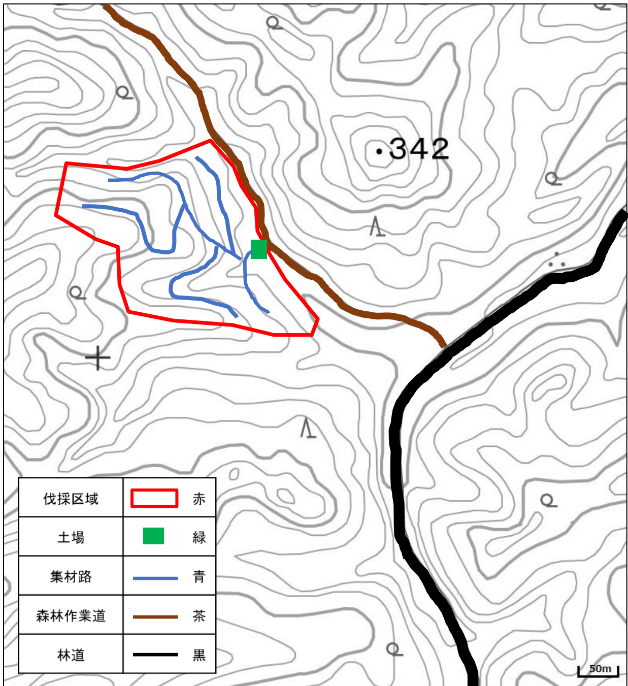
(参考4) 搬出計画図作成例
