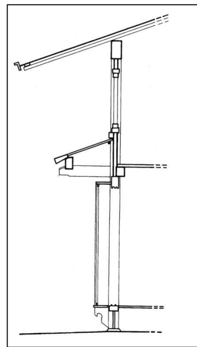
町家矩計図
