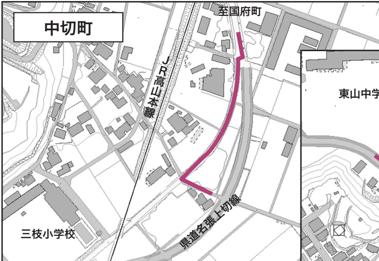
▲公共下水道事業(中切町)
