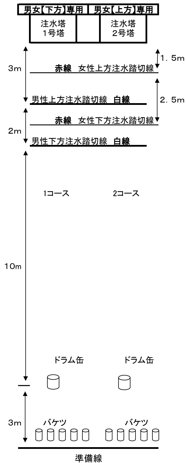
注水要領略図
