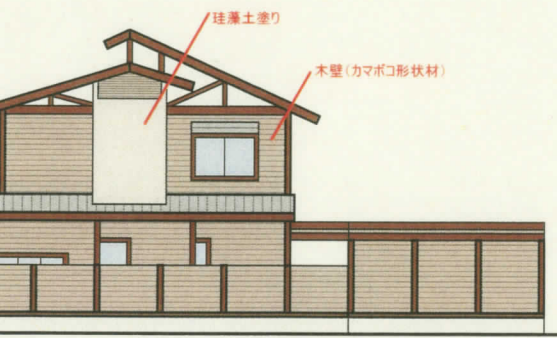
西立面図 1/200
