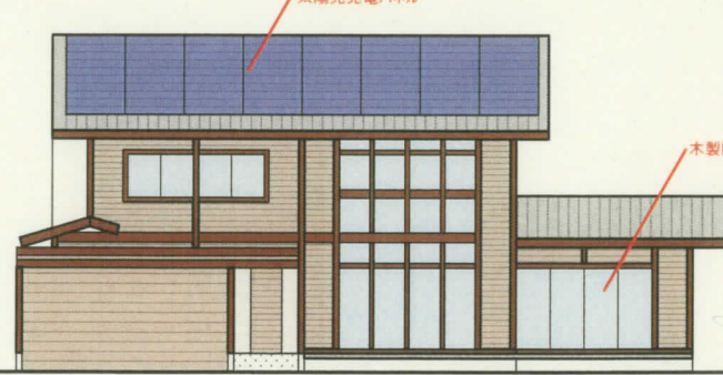
南立面図 1/200
