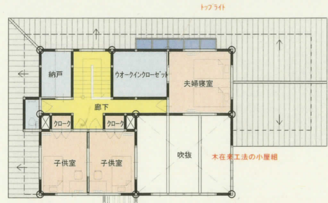
2階平面図 1/200
