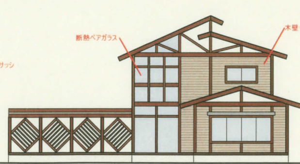
東立面図 1/200
